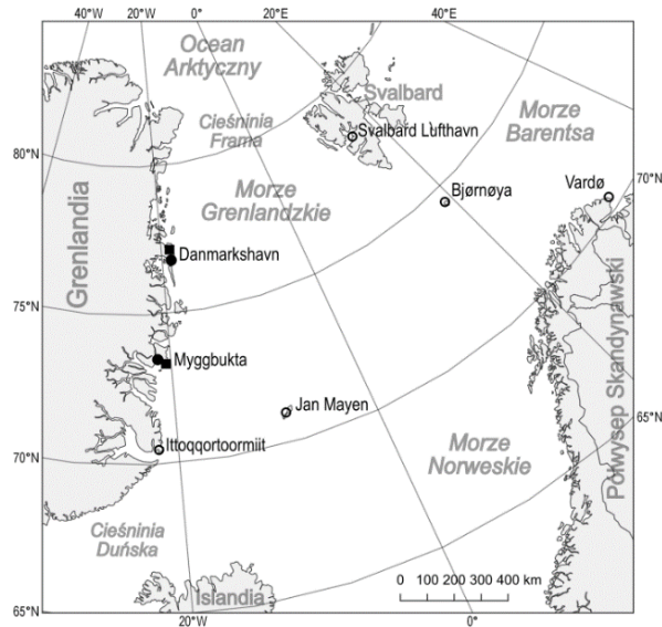
Rycina 1. Położenie stacji meteorologicznych na obszarze Północnego Atlantyku, które zostały użyte w niniejszym opracowaniu. Wypełnione kropki oznaczają stacje z danymi obserwacyjnymi, na podstawie których utworzono rozszerzoną serię temperatury powietrza dla NE Grenlandii. Natomiast kwadraty oznaczają najbliższe punkty gridowe z Reanalizy Dwudziestowiecznej (wer. 20CRv2c).
