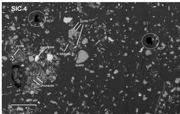
Rycina 2. Obraz elektronów wtórnie rozproszonych (SEM) próbki residuum z lodowca Storebreen (SIC 4); cząstki czarnego węgla (black carbon particles, BCP) zakreślono kółkiem. Strzałkami pokazano ziarna magnetytu, pirytu, skalenia i kwarcu.
