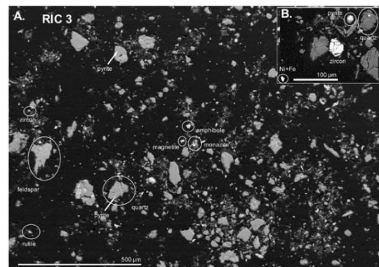
Rycina 3. Obraz elektronów wstecznie rozproszonych (BSE) próbki residuum z lodowca Recherchebreen (RIC 3). W części A widoczne ziarna monacytów. W części B widoczna jest faza Fe-Ni (mikrometeoryt?) oraz duże ziarno cyrkonu.
