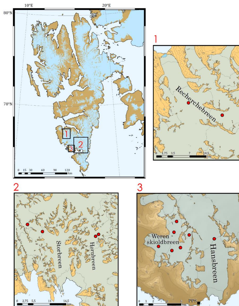
Rycina 1. Lokalizacja obszaru badań (1,2,3) oraz miejsca pobierania rdzeni (czerwone kropki) do badań pyłów eolicznych.
