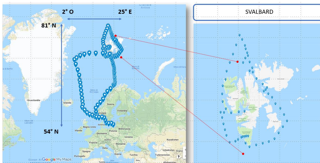
Rycina 1. Rejon badań objęty pomiarami podczas rejsu AREX 2018.
